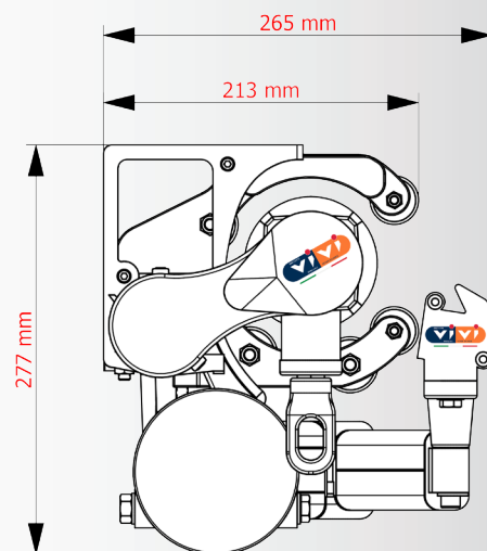
Vista BQ 300 con Reggirullo Tipo 2:
