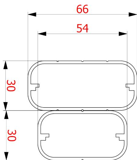
Sezione Profili Braccia Serie 300:
