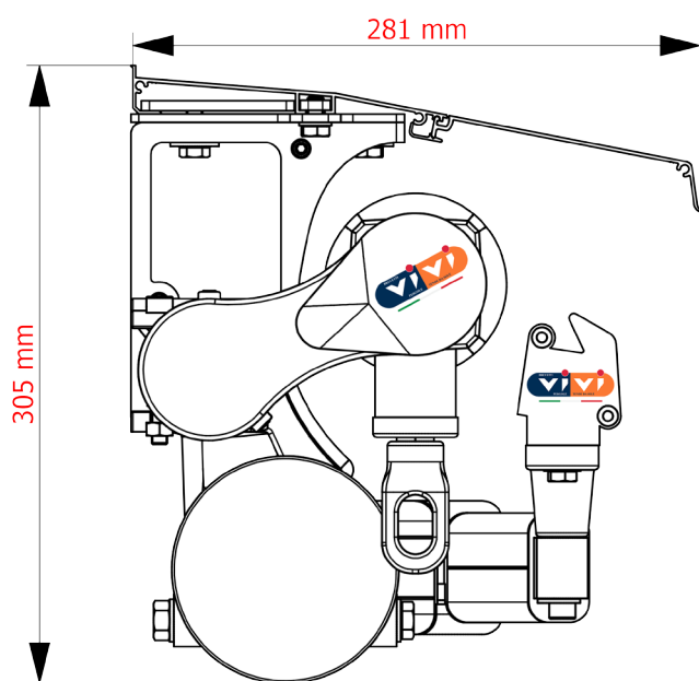
Vista BQ 300 con Tettuccio in Estruso:
