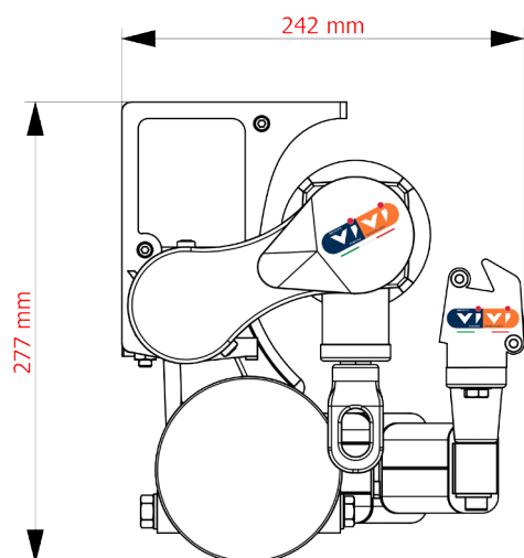
Vista BQ 300 con Tettuccio in Estruso:
