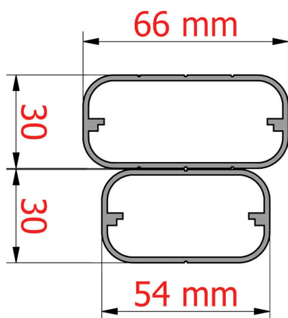
Sezione Profili Braccio Serie 300:
