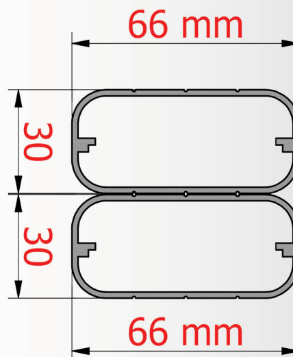
Sezione Profili Braccio Serie 350:
