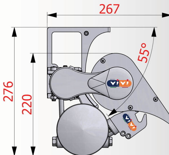
Vista Laterale Inclinata a 55°:
