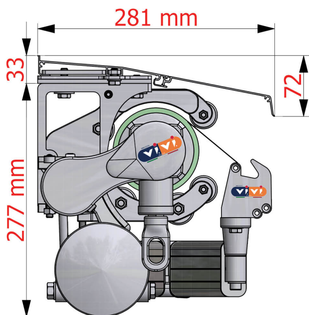
Vista con Tettuccio in Estruso:
