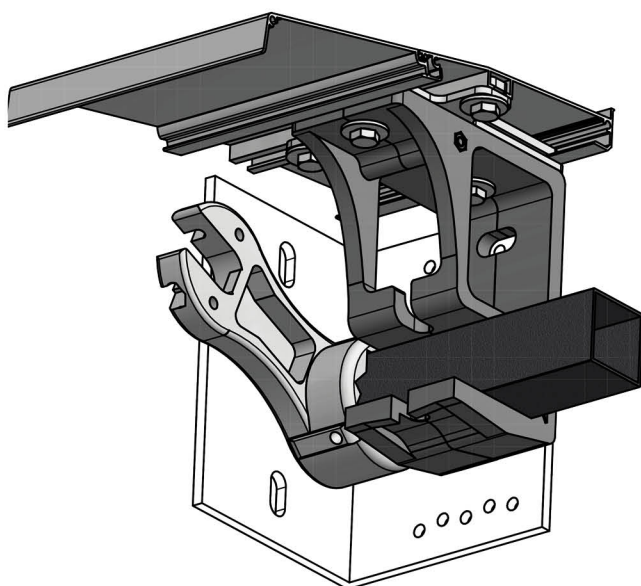
Staffa Speciale per Installazione in Nicchia con Tettuccio:
