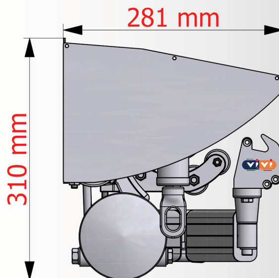
Vista con Tettuccio in Estruso con Tappi Lateral:
