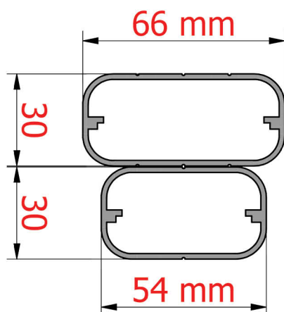
Braccio Serie 300 Sporg. fino a 275 cm
