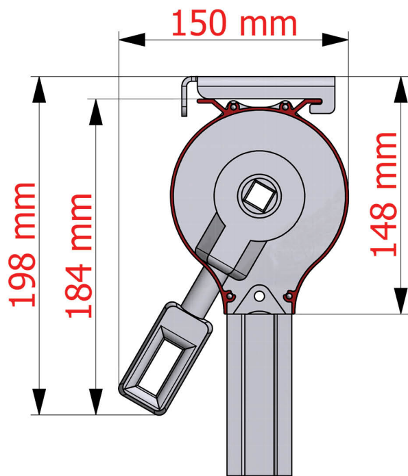
Staffa per la posa della Guida 40 x 40 in Facciata Tipologia 1:
