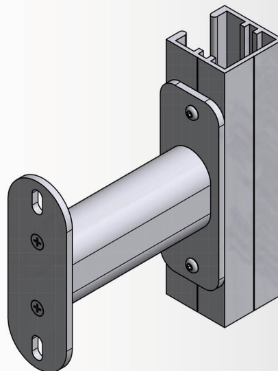
Attacco Guida Tipo 2:
