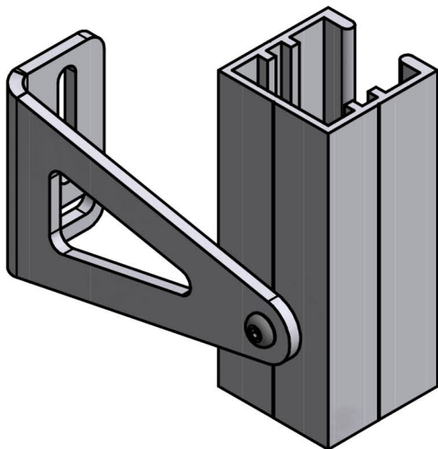
Attacco Guida Tipo 1:
