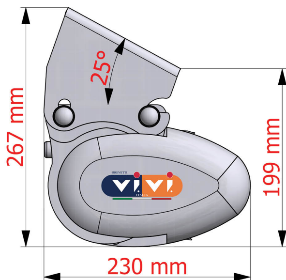
Staffa Speciale per Soffitto o Parete Inclinata 25°:
