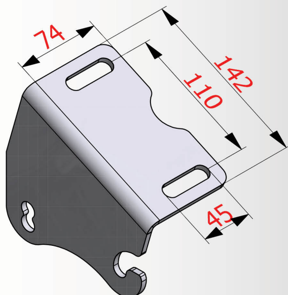
Staffa Speciale per Soffitto o Parete Inclinata 25°:
