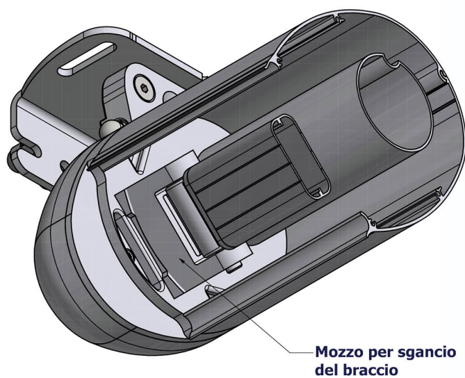
Vista Interna Sezione Maxi Box: (Sgancio del Braccio dalla Struttura)
