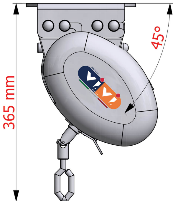
Vista Laterale Maxi Box con Motore con Argano H:
