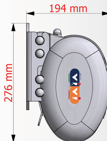
Ingombri Tenda Posa a Parete:
