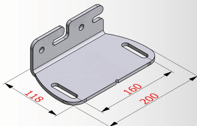
Staffa Installazione Maxi Box 2 Braccia:
