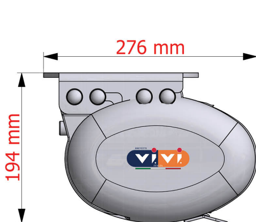
Ingombri Tenda Posa a Soffitto:
