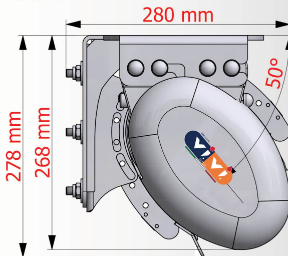
Ingombri Tenda Posa a Soffitto:
