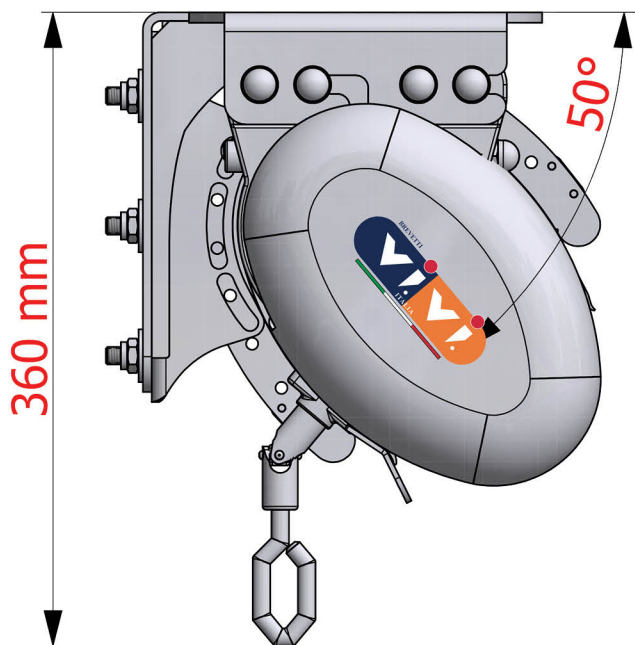
Vista Laterale Maxi Box con Motore con Argano H:
