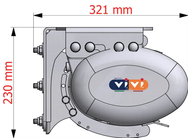
Ingombri Tenda Posa a Soffitto:
