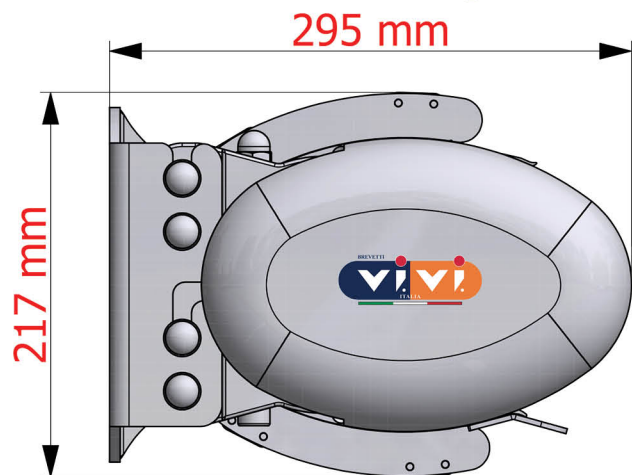
Ingombri Tenda Posa a Parete:
