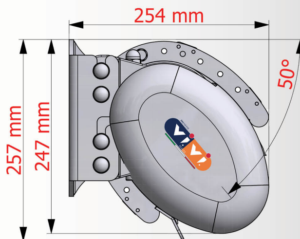
Ingombri Tenda Posa a Parete:
